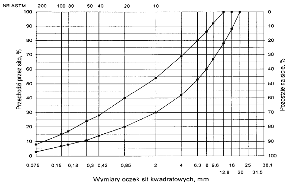
Rys. 1. Krzywe graniczne uziarnienia mieszanki mineralnej BA od 0 do 16 mm do warstwy wiążącej drogi o obciążeniu ruchem KR1
