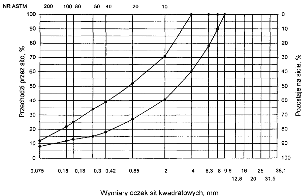
Rys. 1. Krzywe graniczne uziarnienia mieszanki mineralnej BA od 0 do 16mm, do warstwy ścieralnej nawierzchni drogi o obciążeniu ruchem KR1
